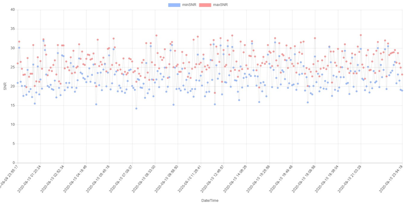
FM SNR chart
